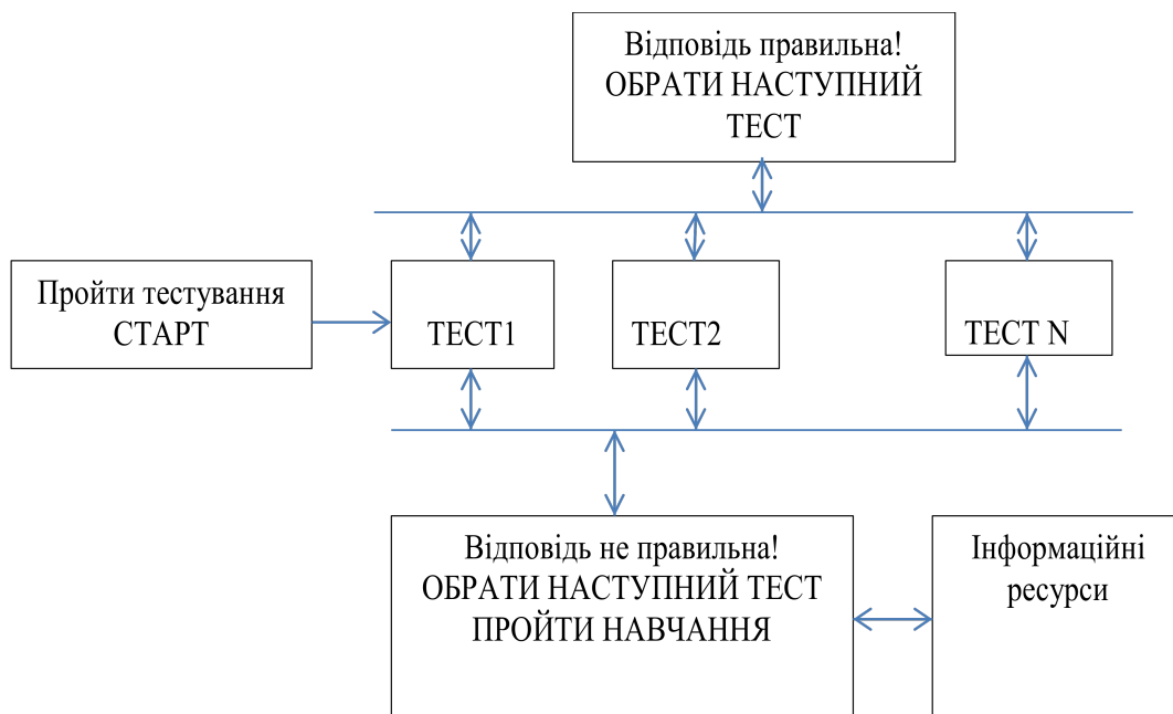
Рис.1. Частина схеми алгоритму побудови тестових завдань
